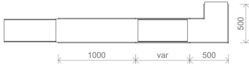
BOVENAANZICHT
