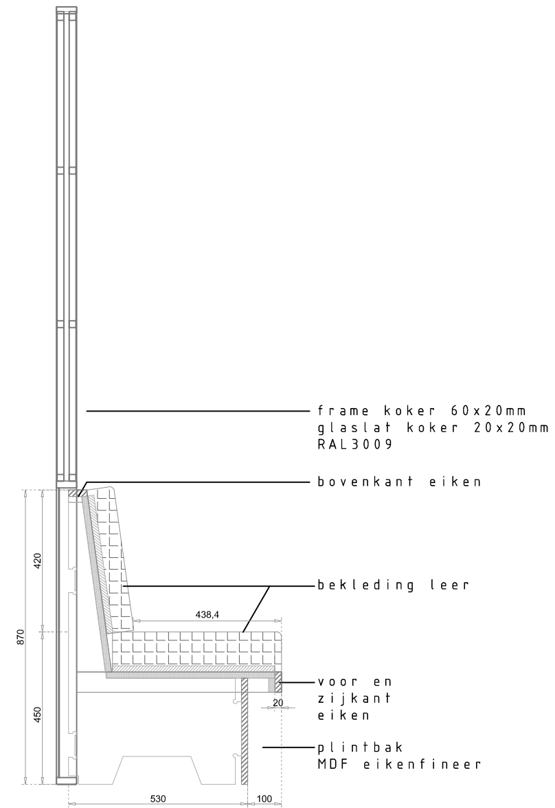
D o o r s n e d e
