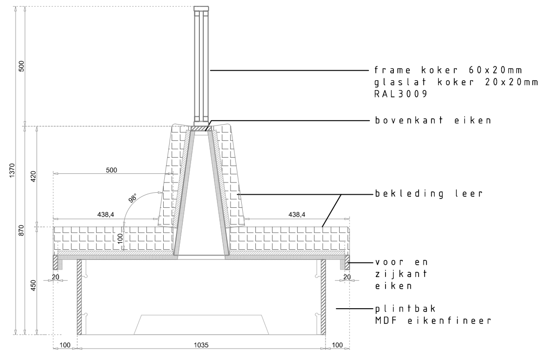
Doorsnede
