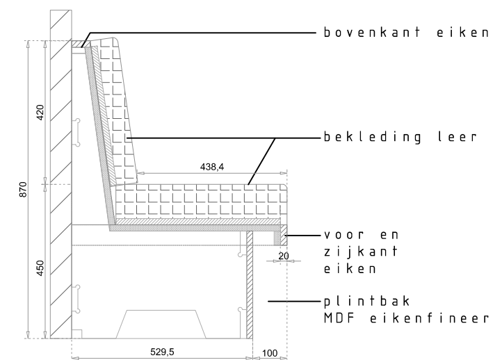
D o o r s n e d e
