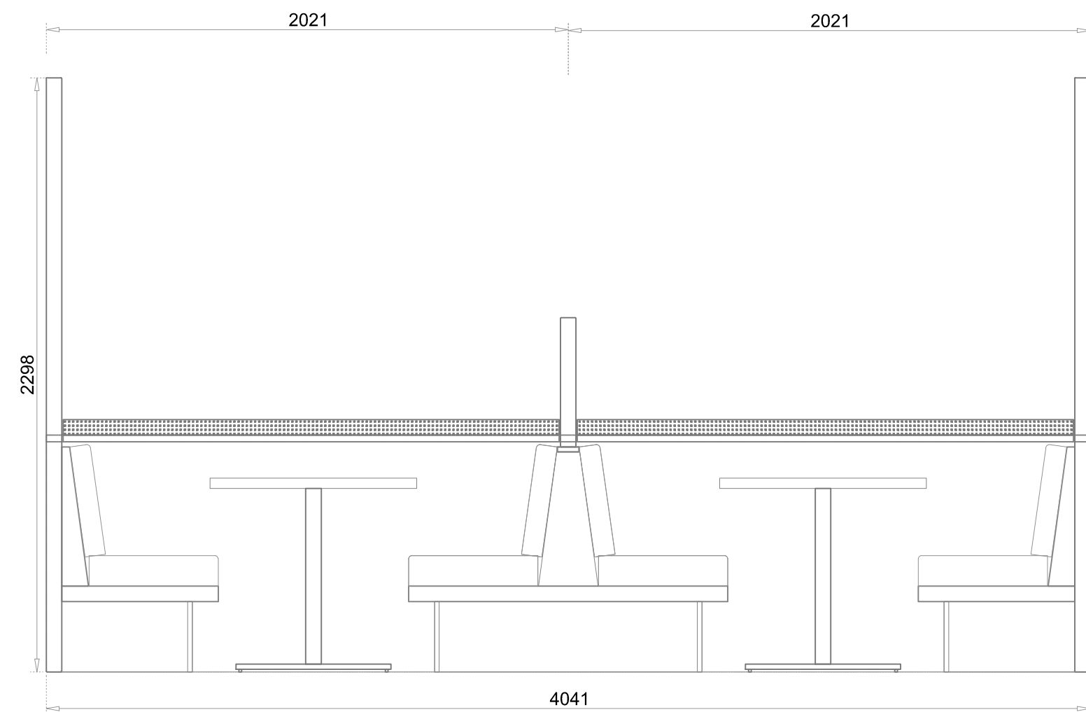
Zijaanzicht
